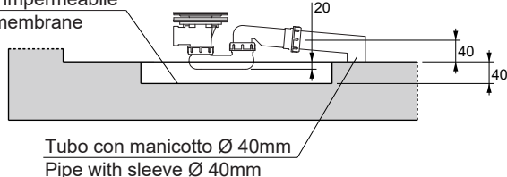
S2: SCARICO PIATTO DOCCIA / SHOWER DRAIN
